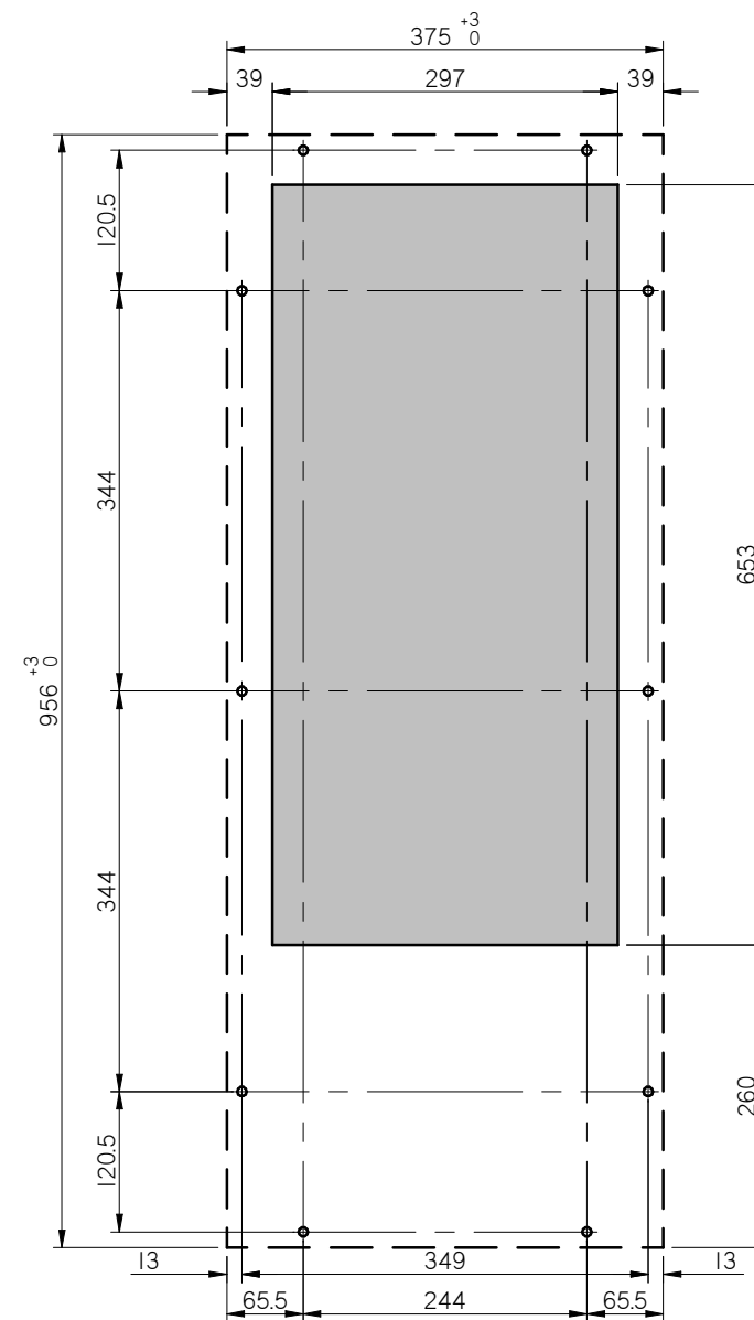
MONTAGGIO ESTERNO EXTERNAL MOUNTING
