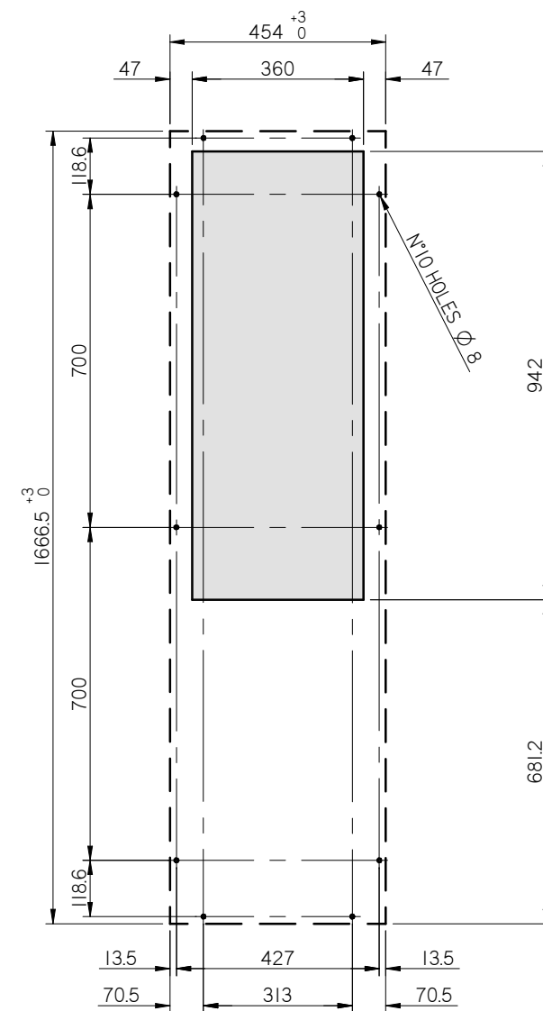
MONTAGGIO ESTERNO EXTERNAL MOUNTING
