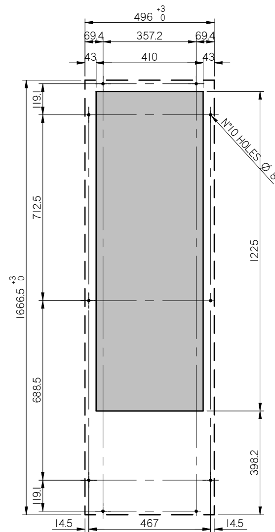
MONTAGGIO ESTERNO EXTERNAL MOUNTING
