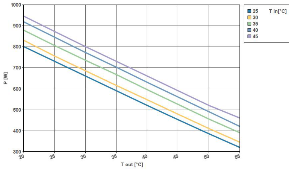
CNx07 230-1-60Hz
