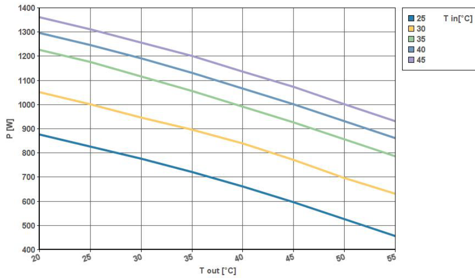
CNx10 230-1-60Hz
