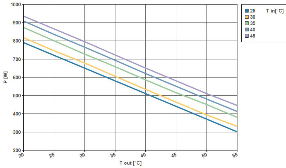
CNx07 230-1-50Hz
