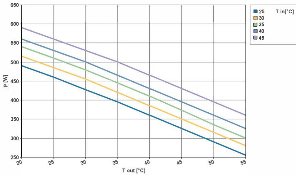
CNx04 400/460-2-50Hz
