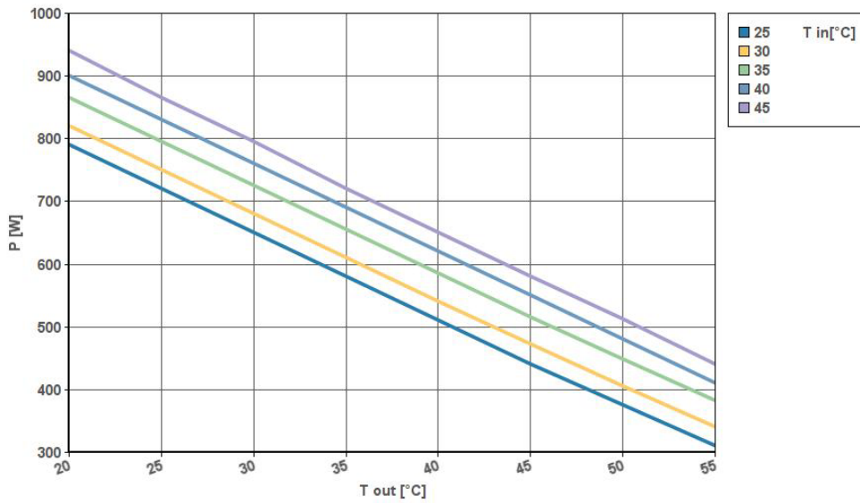
CNx07 400/460-2-60Hz
