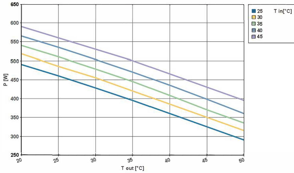
CNx04 115-1-60Hz
