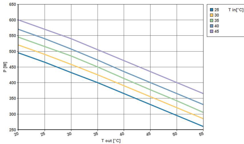
CNx04 230-1-50Hz
