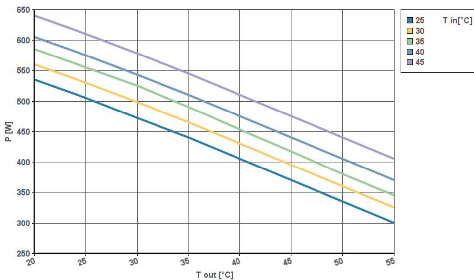
CNx04 230-1-60Hz
