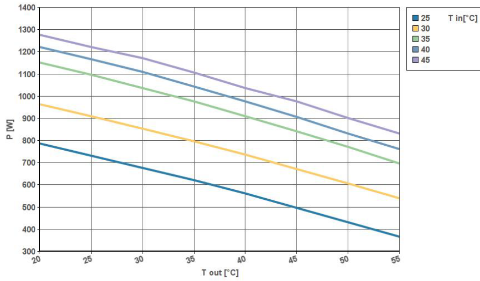
CNx10 230-1-50Hz
